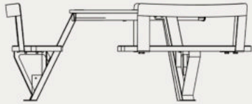
D230*45/77
